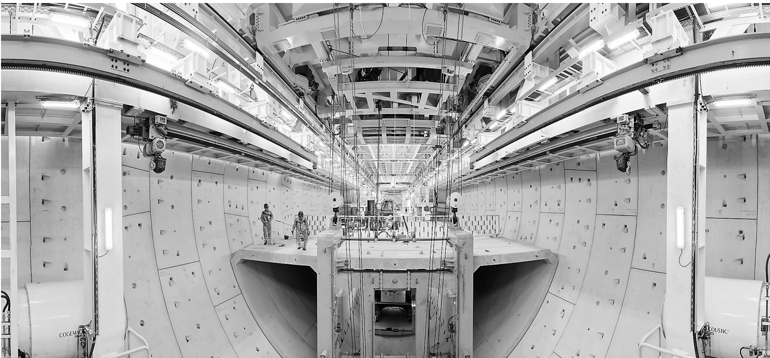
12月7日在江苏省南通市海门区拍摄的海大长江隧道工程盾构掘进施工现场。近日，海大长江隧道右线隧道盾构掘进突破3000米，完成总掘进任务的近三分之一。
