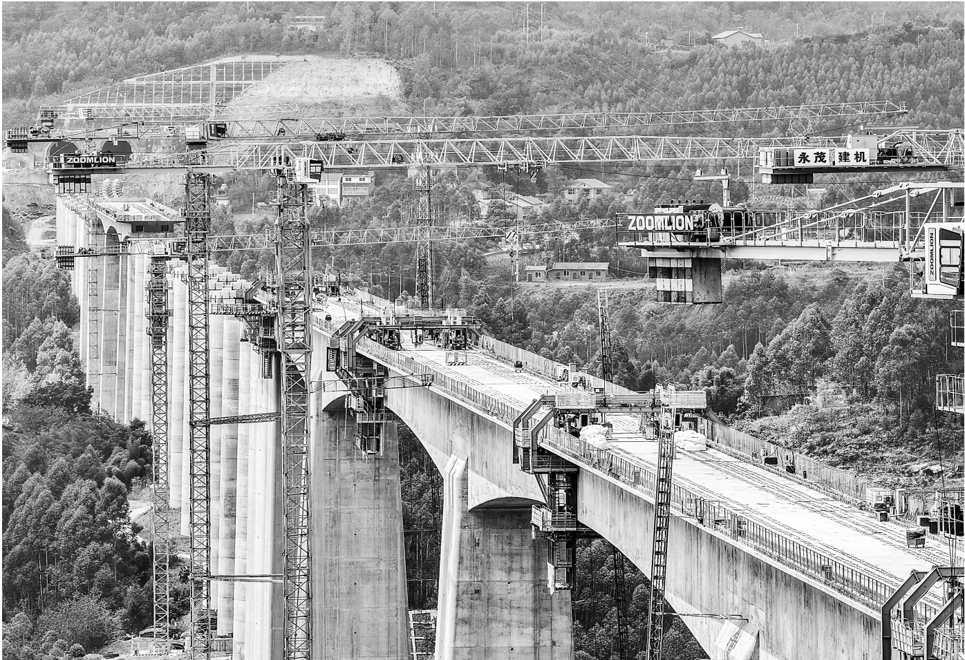
9月1日，由中国铁建大桥局承建的新建重庆至万州高速铁路（渝万高铁）蔡家沟双线特大桥顺利合龙。图为渝万高铁蔡家沟双线特大桥建设现场。新华社记者 唐奕
