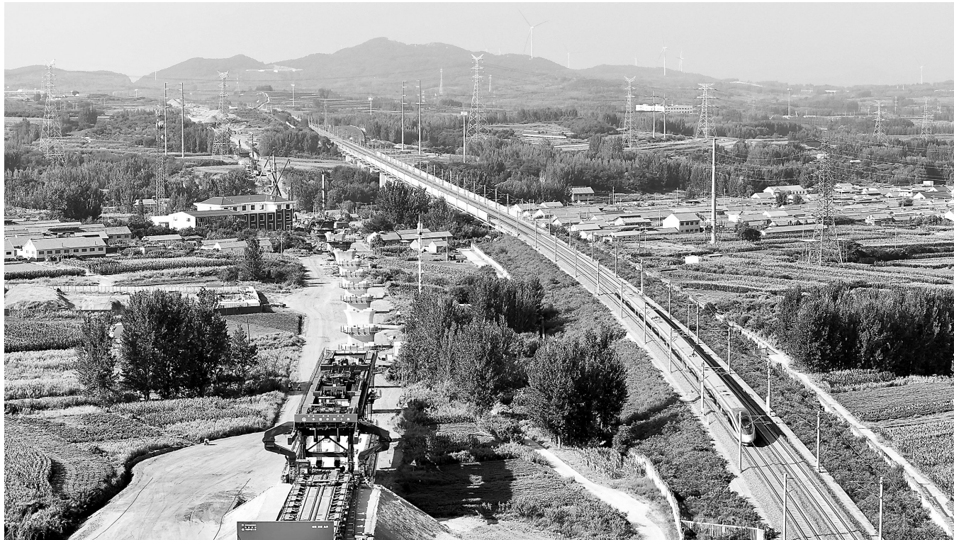
8月22日,潍(坊)宿(迁)高铁至青岛连接线1标段首榀箱梁架设成功,标志着潍宿高铁至青岛连接线全部4个标段进入全线架梁施工阶段。图为潍宿高铁至青岛连接线1标段沙河中村特大桥施工现场。
