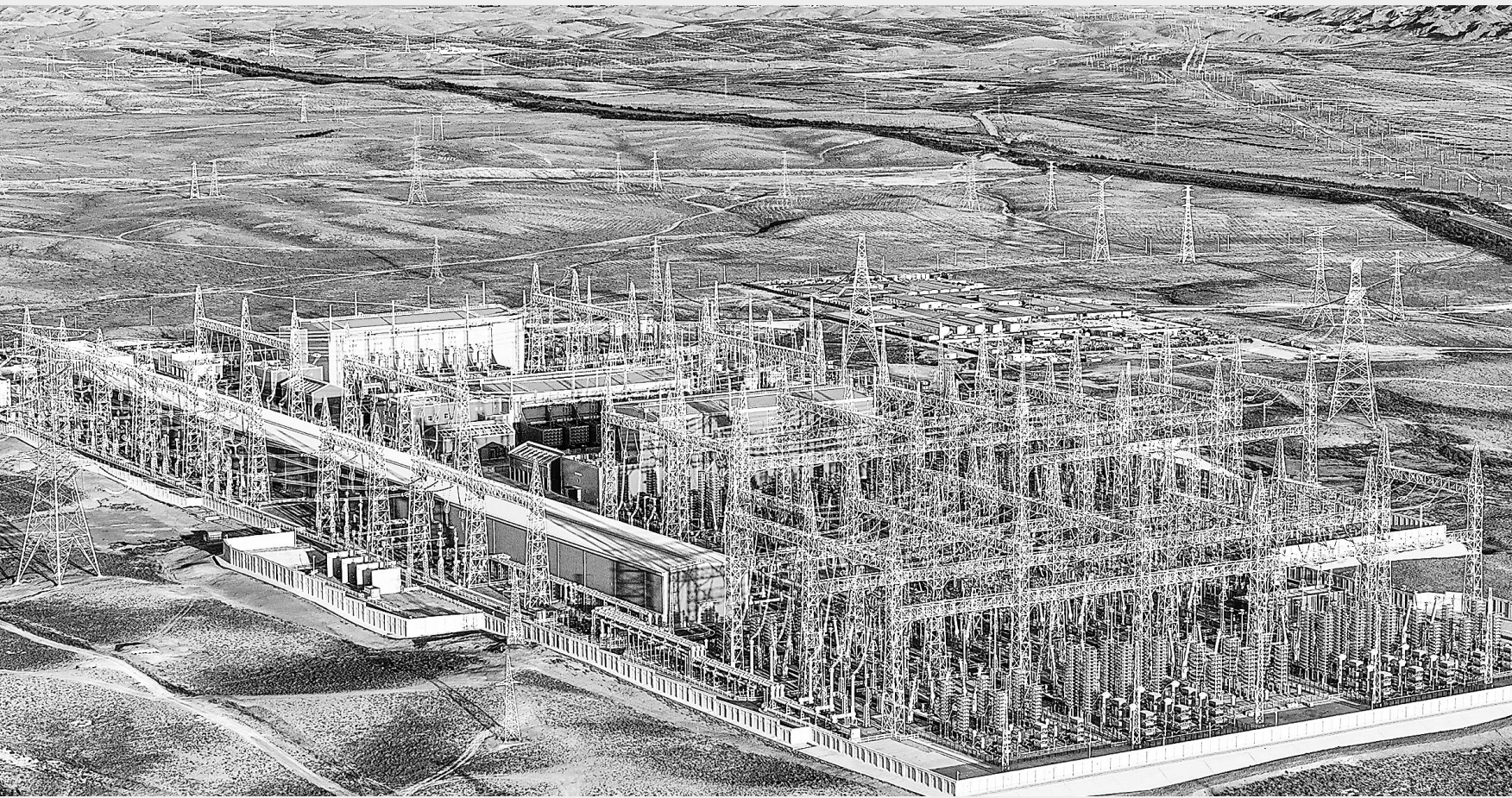
这是8月19日拍摄的“宁电入湘”工程宁夏中卫市中宁换流站。当日,国家电网有限公司宁夏—湖南±800千伏特高压直流输电工程(“宁电入湘”工程)投产送电。作为连接西部新能源富集区与中部负荷中心的重要通道,工程起于宁夏回族自治区中卫市中宁换流站,途经甘肃、陕西、重庆、湖北,止于湖南省衡阳市衡阳换流站,线路全长1616公里。
