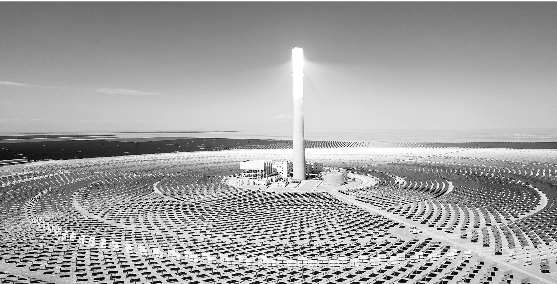
近日,在金塔多能互补基地“10万千瓦光热+60万千瓦光伏”项目现场,连片的光伏板和光热定日镜阵列有序排布。据了解,该项目每年可向电网输送清洁电力14.5亿千瓦时,减少二氧化碳排放量约136万吨。
