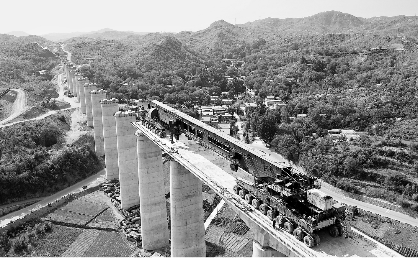
5月27日,雄(雄安新区)忻(忻州市)高铁河北段工程正在按照建设节点要求高标准、高质量施工。雄忻高铁建成通车后将服务于京津冀城市群和晋中城市群的旅客交流,有效疏解环北京地区的客运压力。图为工人在雄忻高铁河北段站前四标建设工地施工。
