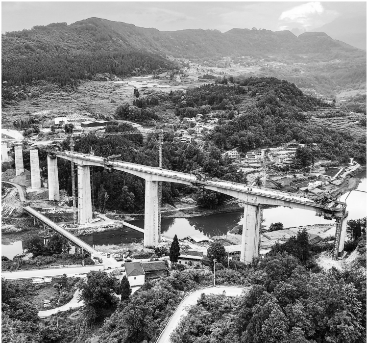
这是5月3日拍摄的渝万高铁汝溪河双线特大桥建设现场。5月4日凌晨,由中铁十八局承建的新建重庆至万州高速铁路(渝万高铁)汝溪河双线大桥全桥顺利实现合龙。新华社记者 唐奕
