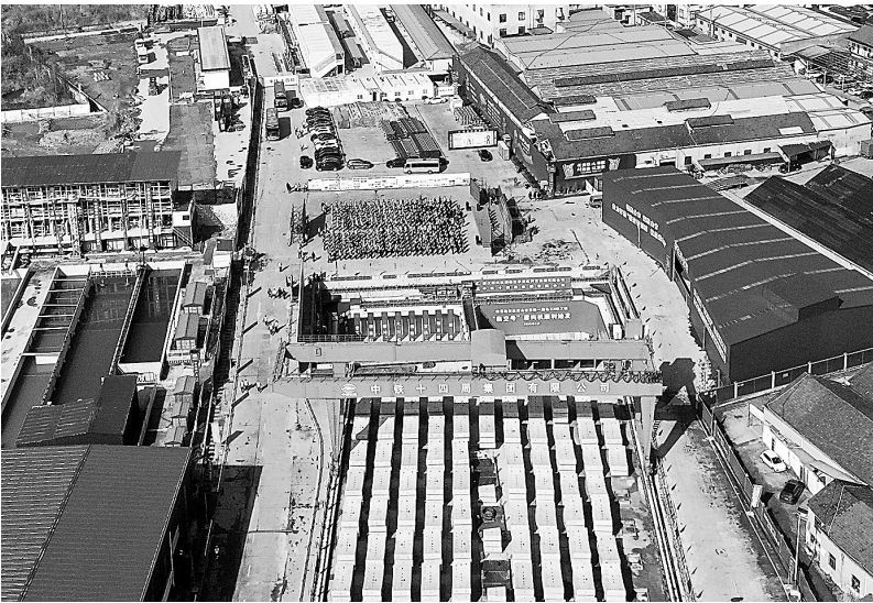
2月28日在浙江省绍兴市柯桥区拍摄的群贤路西延萧山南秀路一期Ⅱ标工程盾构施工现场。据了解,群贤路西延至萧山南秀路项目是绍兴市全面融入“长三角地区一体化发展”的基础工程,计划于2026年建成。 新华社发
