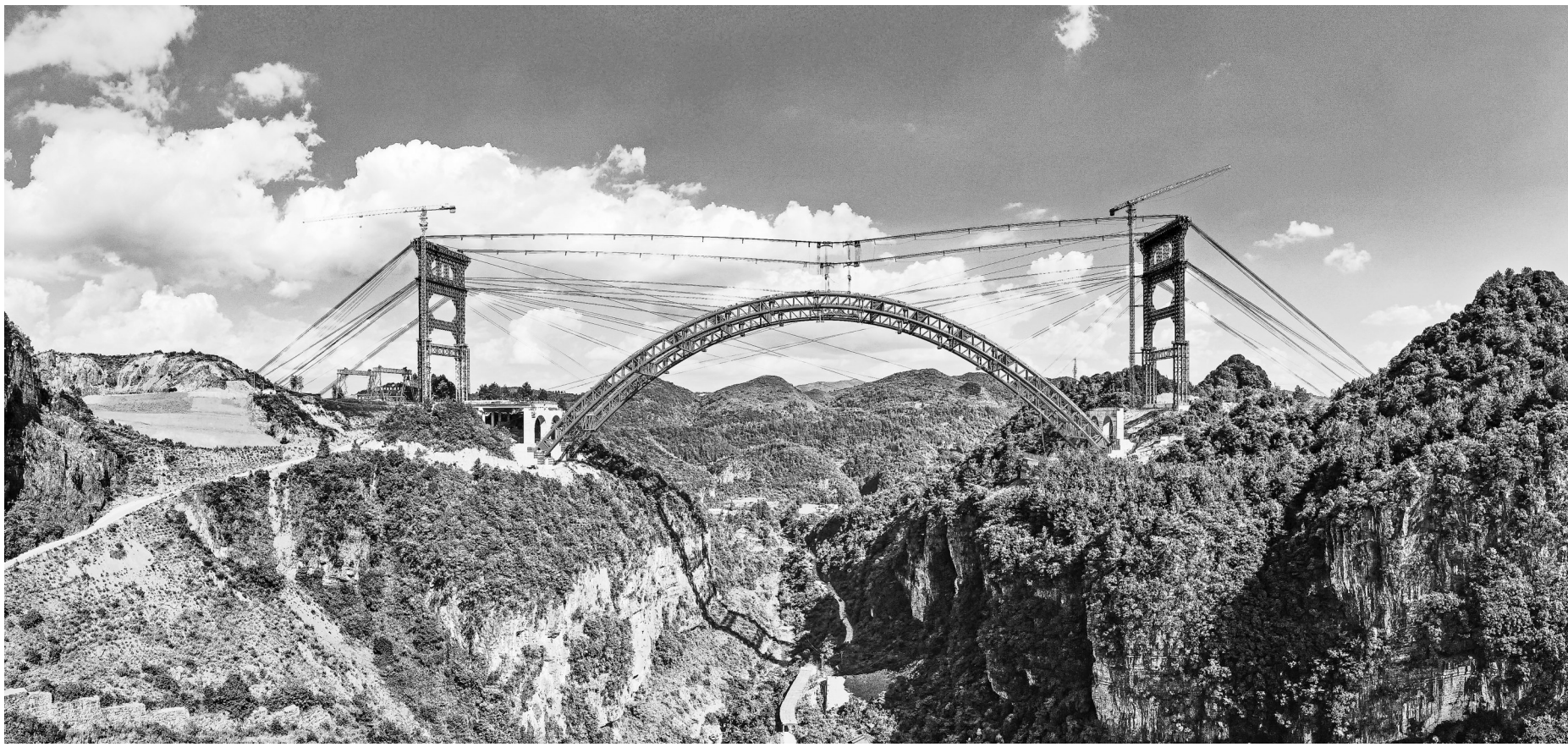
8月21日，由贵州桥梁集团承建的贵阳至平塘高速公路马场河特大桥主拱顺利合龙。马场河特大桥位于贵州省贵定县盘江镇马场河村，大桥全长381.5米、主跨260米，桥面设计为双向六车道，是G7522贵阳至北海高速公路贵阳至平塘段控制性工程。
