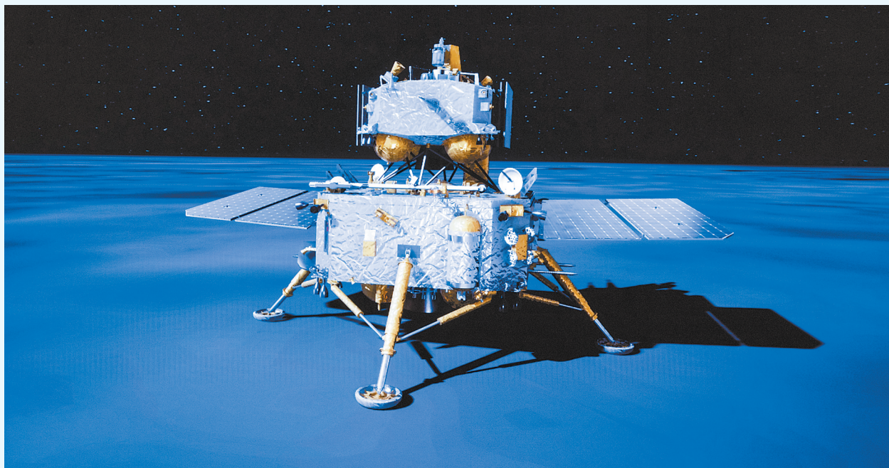
6月2日在北京航天飞行控制中心屏幕上拍摄的嫦娥六号着陆器和上升器组合体着陆月球背面的模拟动画画面。新华社发
