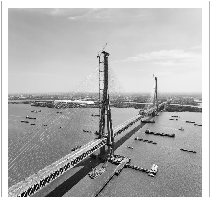
5月29日,常泰长江大桥主航道桥最后一节钢桁梁——合龙段钢桁梁顺利吊装到位,拉开主桥合龙的序幕,预计6月上旬完成合龙,实现全桥贯通。 新华社发
