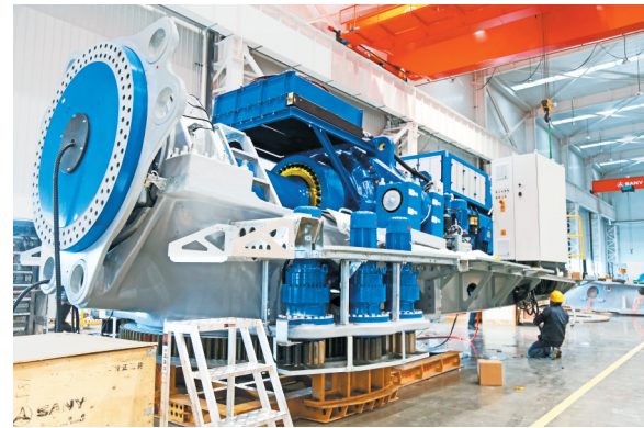
近日，在位于庆阳市西峰工业园区的庆阳三一风电智能制造项目生产车间，工作人员忙着组装、检测首台风电机组。该项目于今年4月底建成投产。
