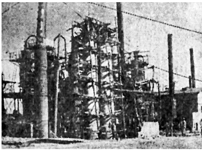
玉门油矿炼油厂改建达布斯裂炼炉。(《甘肃日报》1950年8月23日第3版)
