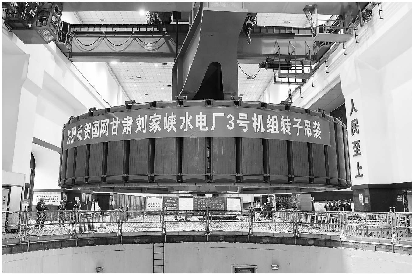
4月25日19时50分,随着重达593.6吨、直径11.69米的发电机转子缓缓吊入机坑,标志着国网甘肃刘家峡水电厂3号机组整机组造工程进入回装关键阶段。新甘肃·甘肃日报通讯员 侯齐
