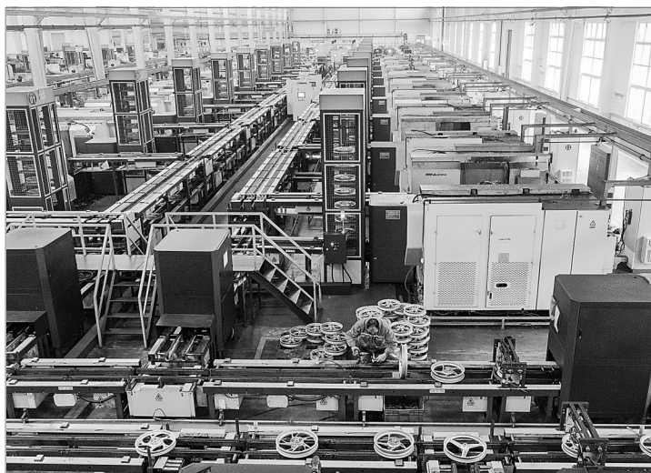
近年来,重庆垫江县通过政策扶持、市场引导、服务推进等有效措施,引导当地摩托车轮胎生产龙头企业产业提档升级。图为近日重庆捷力轮毂制造有限公司的自动化轮毂生产线。新华社发
