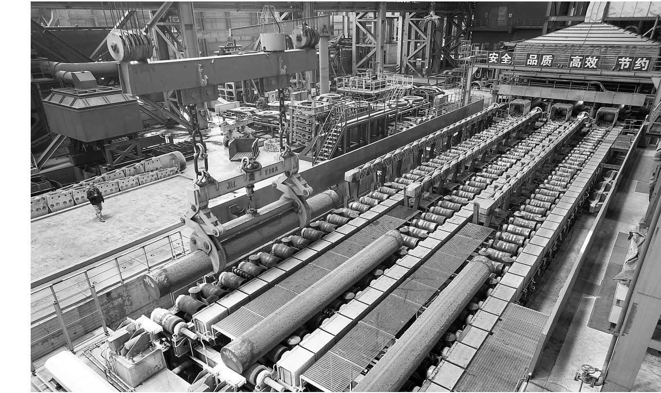
近期,1300毫米粗坯连铸圆坯生产线在河北省承德市营子区的大型特殊钢铁生产企业实现量产,1300毫米粗坯连铸圆坯的量产将逐步改写大厚壁法兰采用钢锭锻造的历史,为我国能源领域大型装备的生产提供重要支撑。
